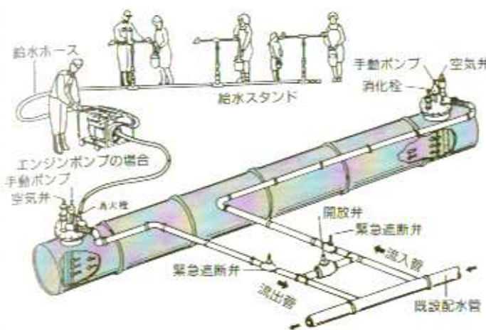
耐震性貯水槽の概要図
