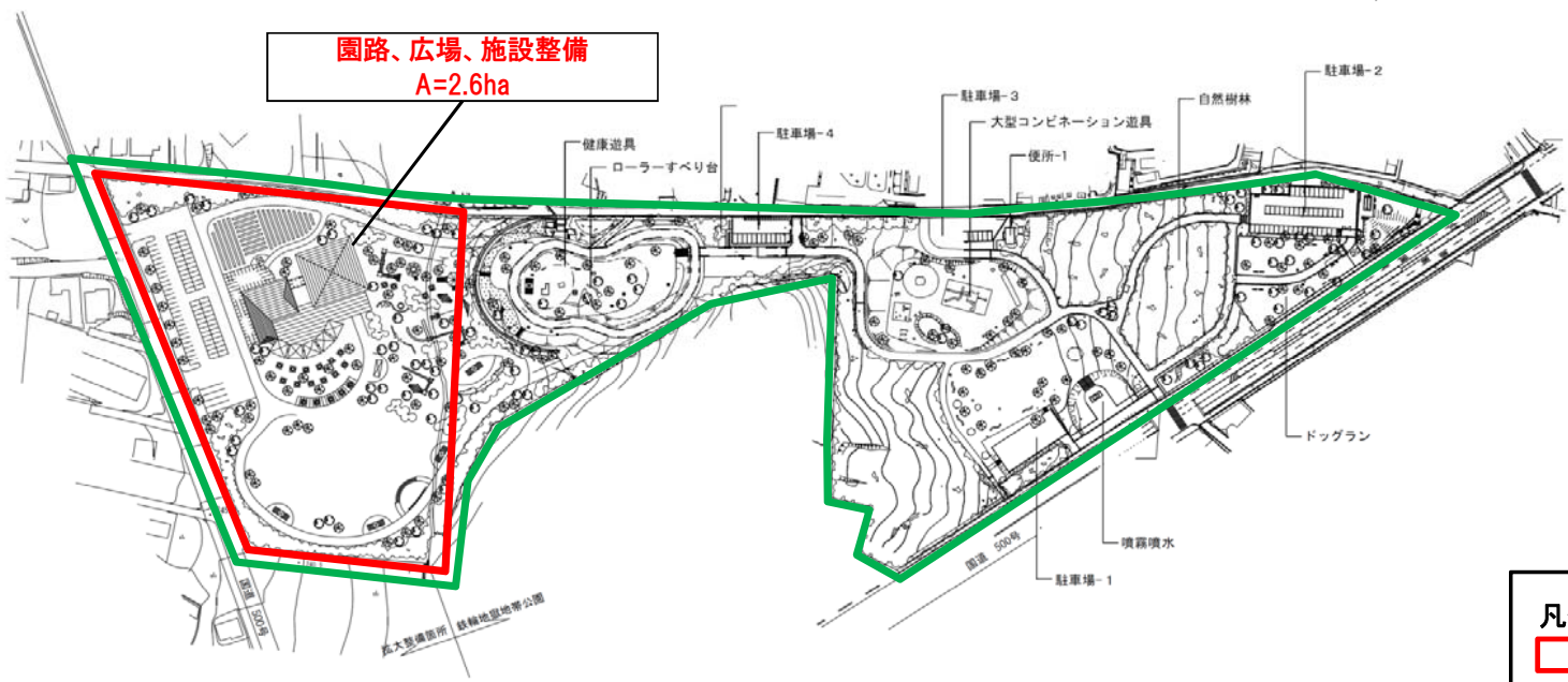
計画平面図
