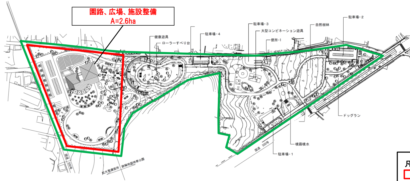
計画平面図
