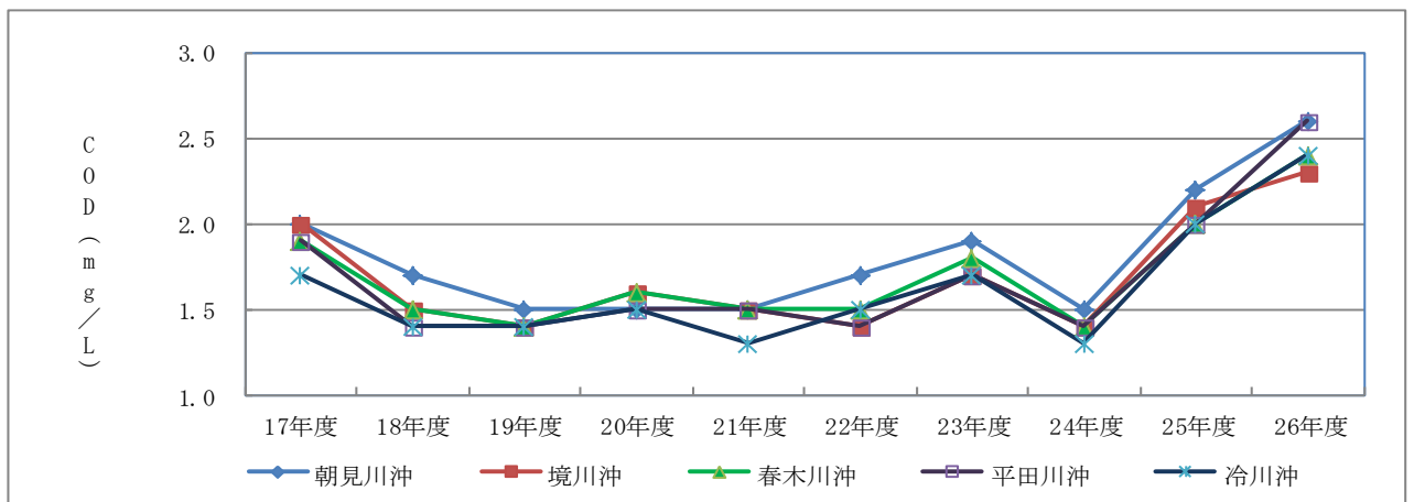
図表 2.16 別府湾地先海域 5 定点の COD 濃度の各年度の経年変化
